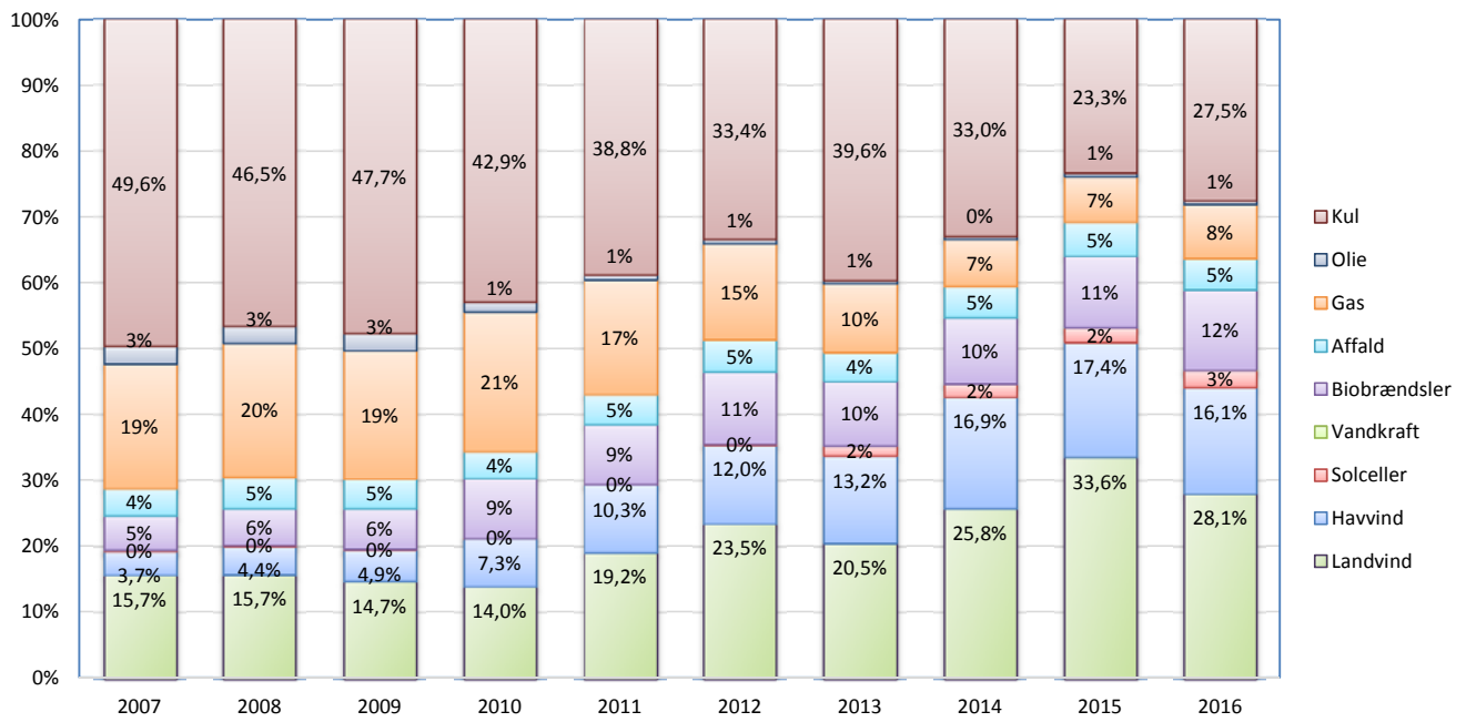
Dansk elproduktions sammensætning fordelt på brændsler (% af nettoproduktion)
